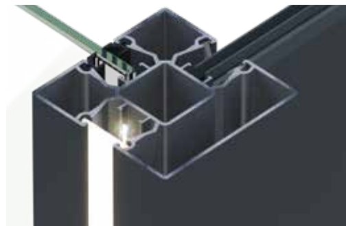
Pfahl mit Alu-Profil, Glasscheibe, LED-Flex-Modul-Streifen und Acrylglas-Pfahlabdeckleiste
