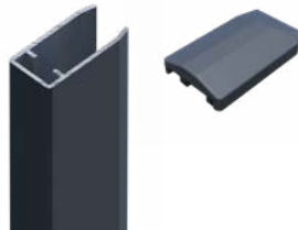
Alu Universalprofil, Anthrazit RAL 7016**, inkl. Abdeckkappe, 50 x 25 x 50 mm, nutzbar als Wandanschluss oder für Eckausbildung am Alu Pfahl
